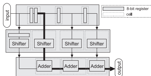
Fig. 5. 4-tap FIR filter.
